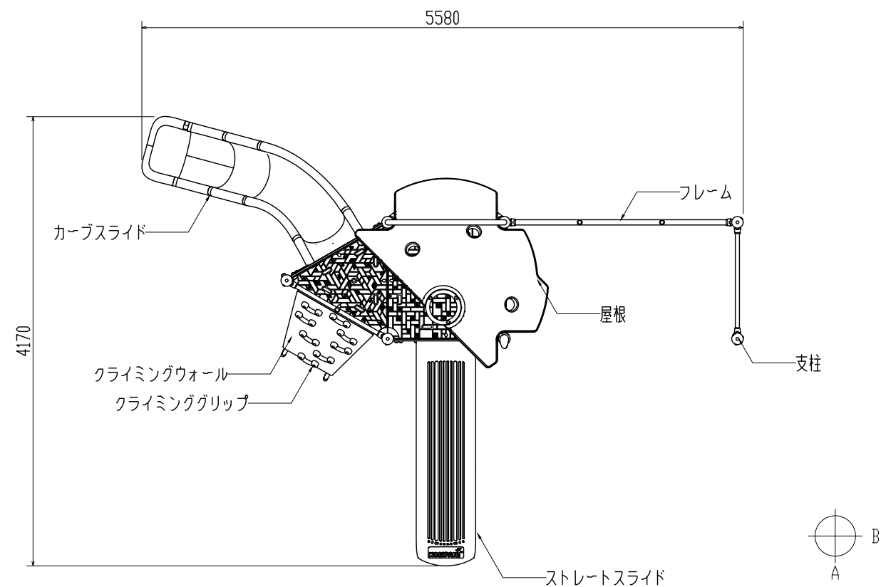
平面图 1/50
