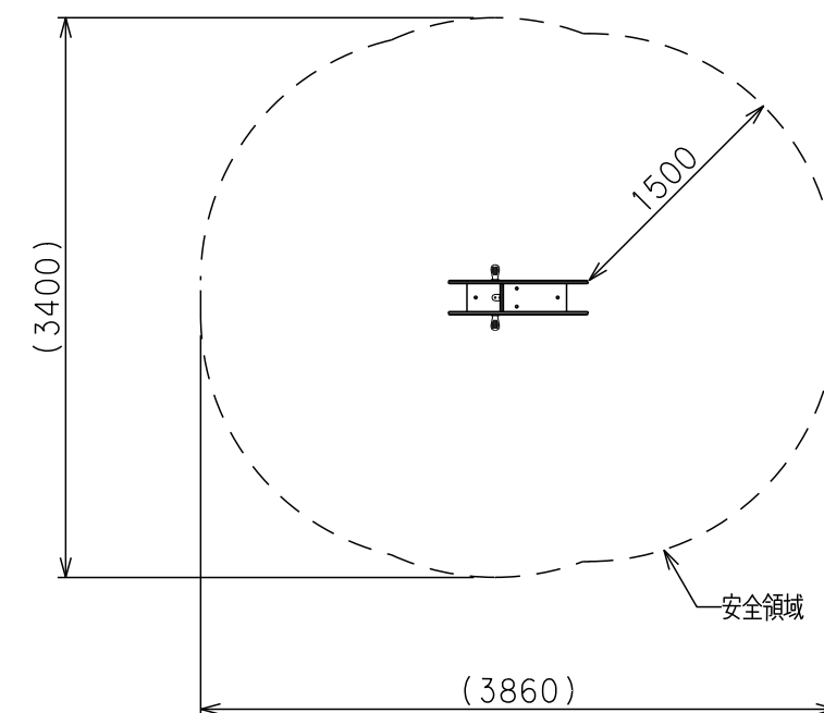
安全領域図 S=1/50
