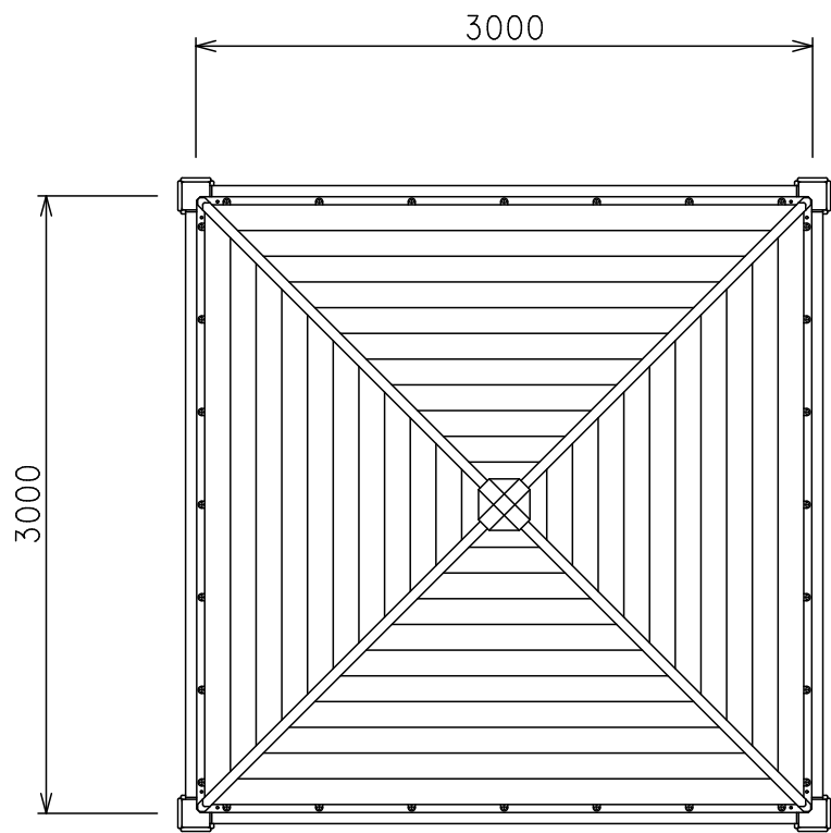
平面図 S=1/40
