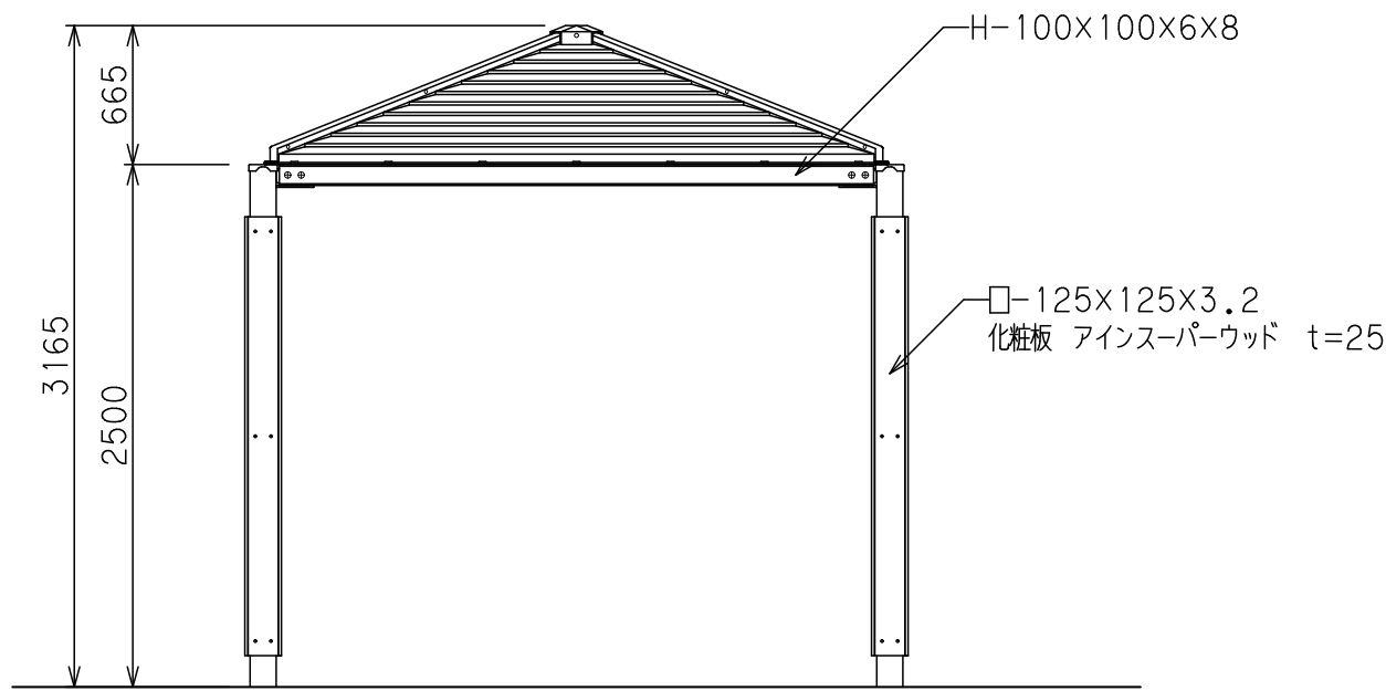
立面図 S=1/40
