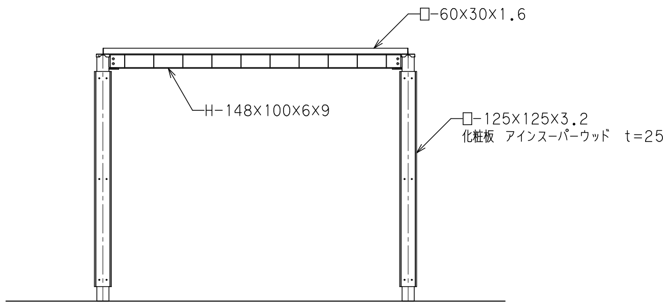
立面図 S=1/40
