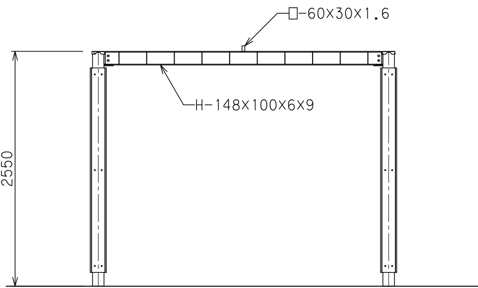
立面図 S=1/40
