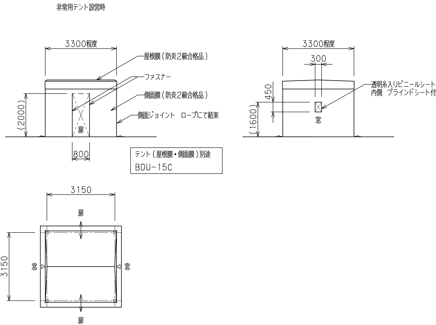
テント詳細図 S=1/100
