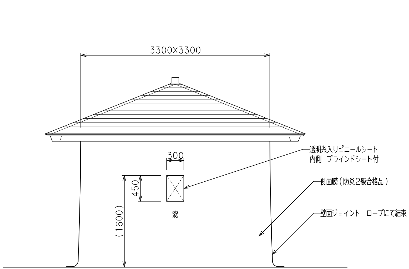
側面図 S=1/40
