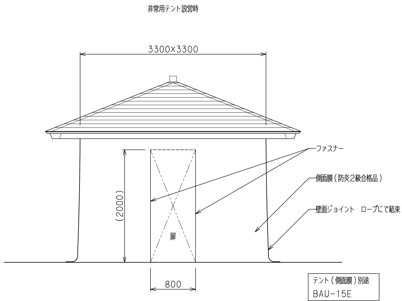
正面 / 背面図 S=1/40
