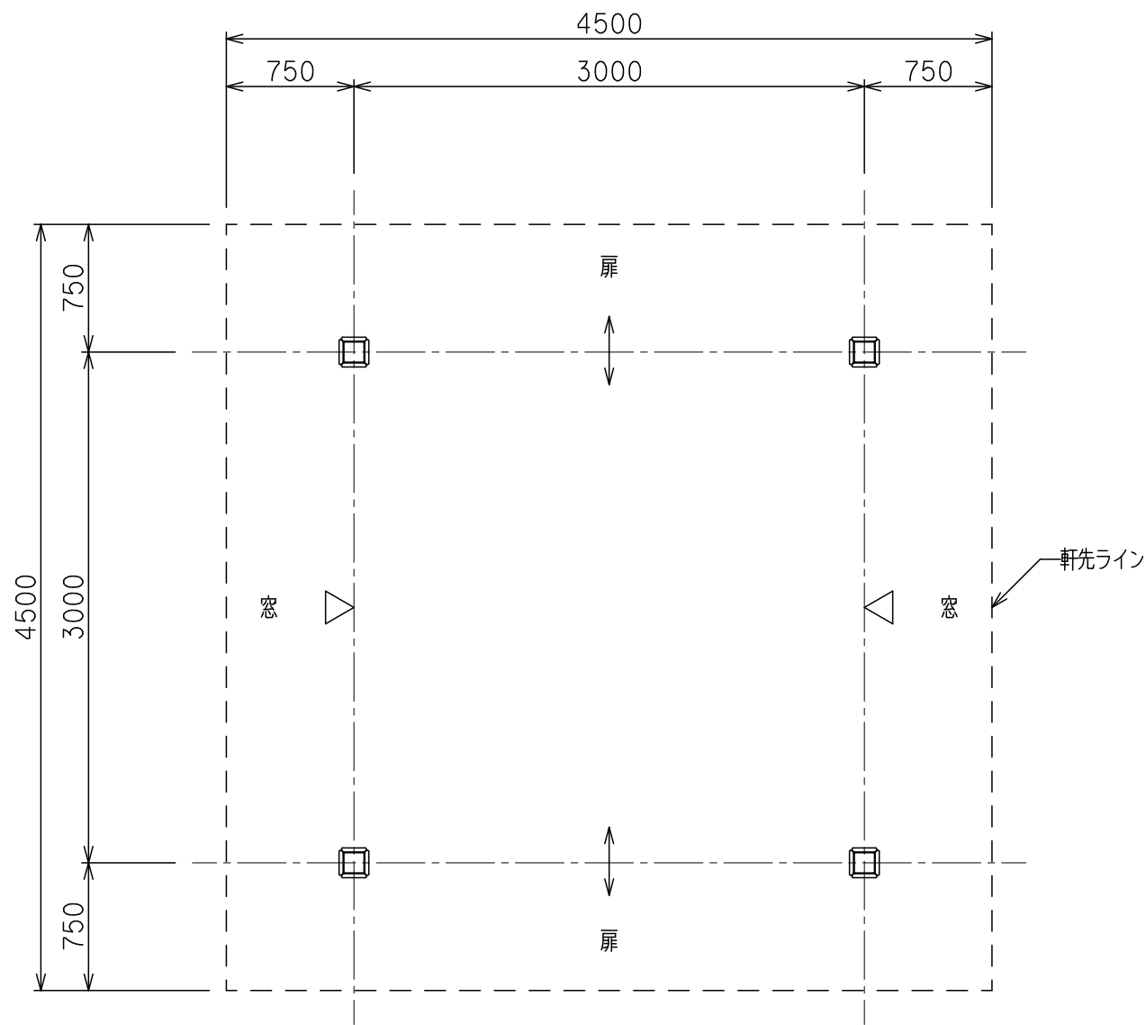
平面図 S=1/40
