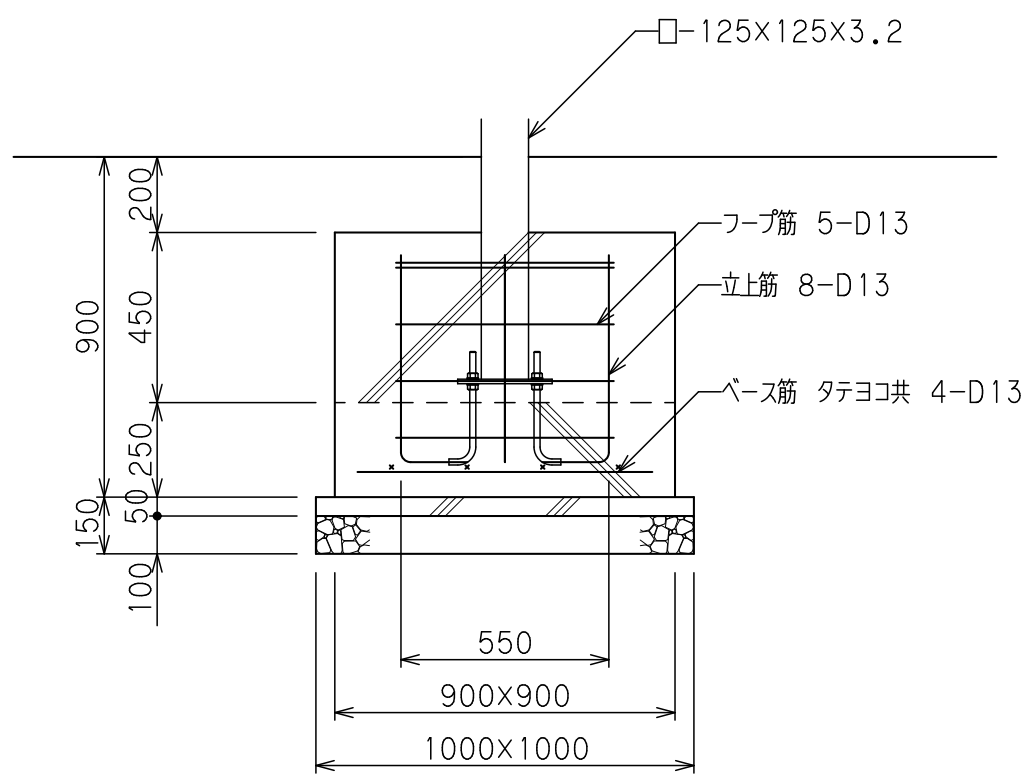
詳細図 S=1/20
