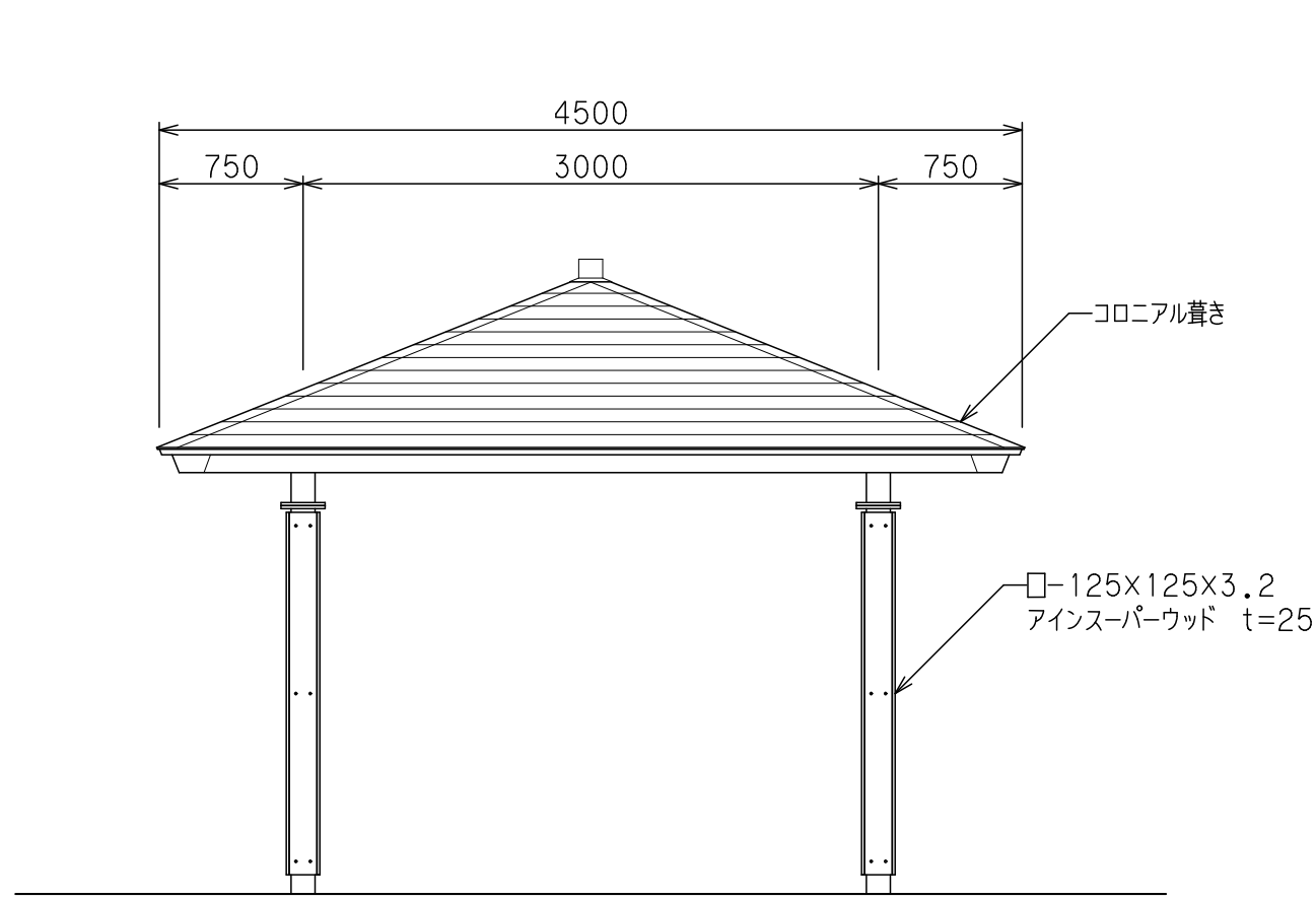
立面図 S=1/40
